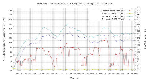
(b) Testfahrt bei -14 bis -19°C
