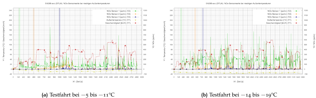
Abbildung 19: Vergleich: NOx-Sensorwerte bei ähnlicher Fahrweise, aber verschiedenen Außentemperaturen
