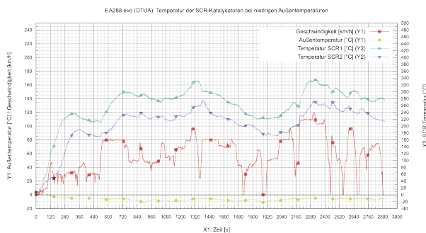
(a) Testfahrt bei -5 bis -11°C
