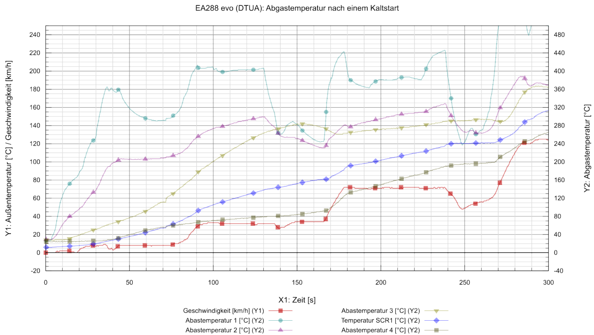
(a) Aufwärmzeit bei -5^{\circ}\text{C}
