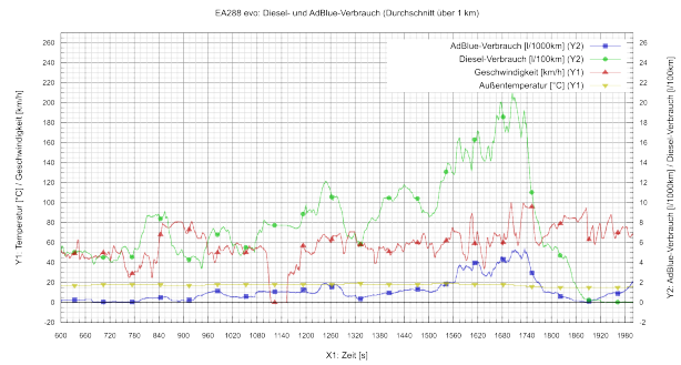
(b) Verbrauch im 1-km-Durchschnitt
