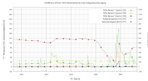
(b) nach Autobahnfahrt
