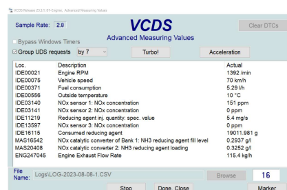
Abbildung 7: Aufnahme mit hoher Ammoniak-Beladung
