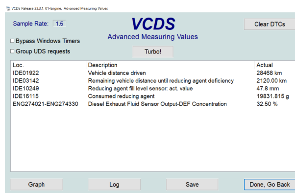
(d) AdBlue-Verbrauch bei 28.468 km
