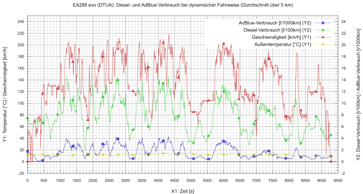
Abbildung 13: Verbrauch bei hoher variabler Geschwindigkeit
