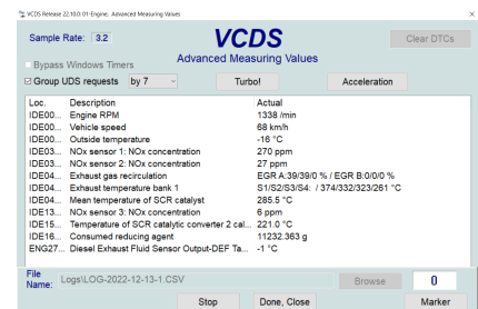
Abbildung 18: Momentaufnahme bei niedrigen Außentemperaturen
