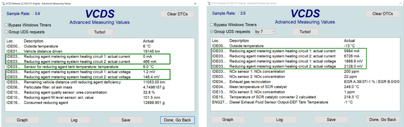
(a) Heizleistung bei +6°C (b) Heizleistung bei -13°C Abbildung 22: Vergleich: Heizleistung im AdBlue-System bei verschiedenen Temperaturen
