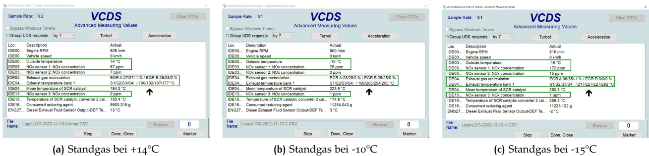
(a) Standgas bei +14°C (b) Standgas bei -10°C (c) Standgas bei -15°C Abbildung 23: Temperaturen im Abgassystem bei Standgas
