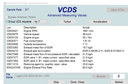
(e) AGR im Stadtverkehr, sehr niedrige Last
