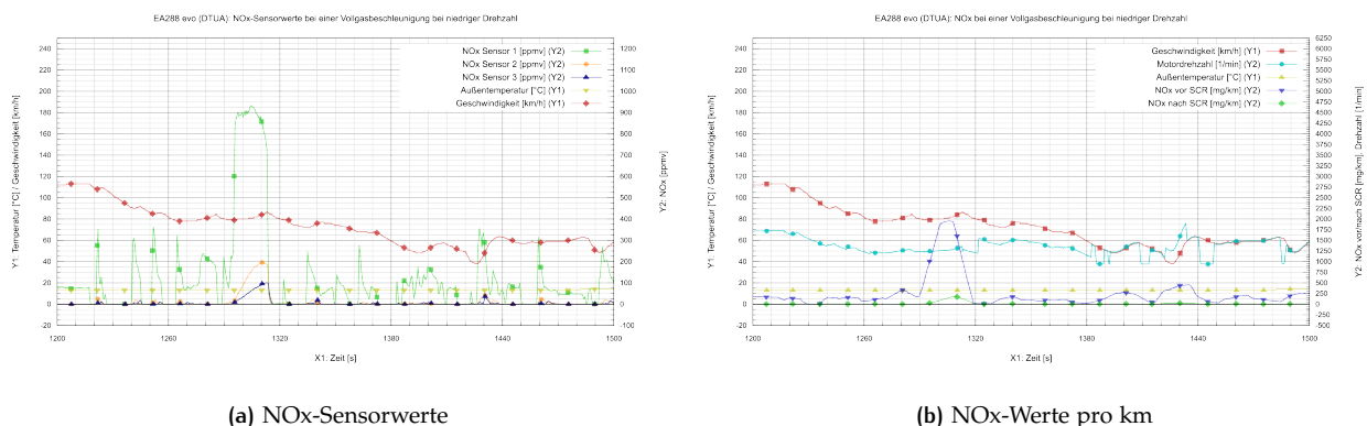
Abbildung 15: NOx-Werte bei einer Vollgasbeschleunigung bei niedriger Drehzahl
