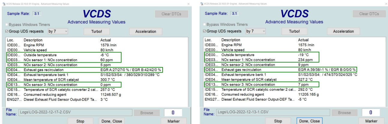
(a) 80 km/h bei -6^{\circ}\text{C} .
