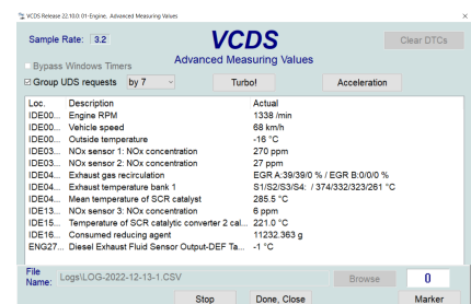
Abbildung 17: Momentaufnahme bei niedrigen Außentemperaturen
