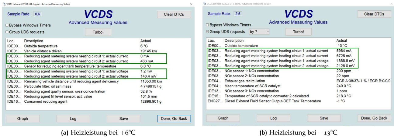
Abbildung 21: Vergleich: Heizleistung im AdBlue-System bei verschiedenen Temperaturen
