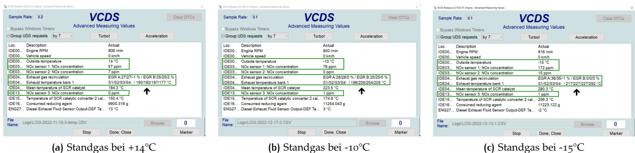
Abbildung 22: Temperaturen im Abgassystem bei Standgas
