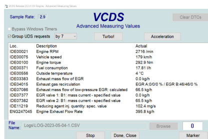
(b) AGR bei 180 km/h, höhere Last
