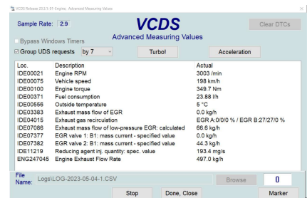
(c) AGR bei 200 km/h, höhere Last
