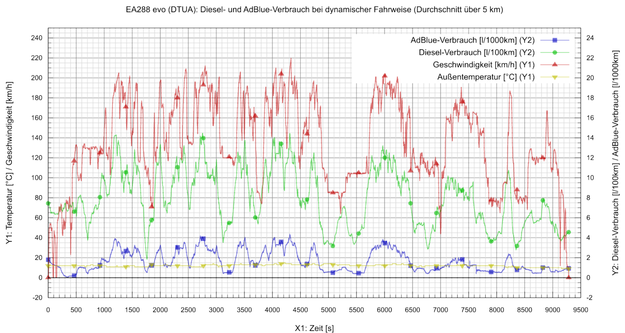
Abbildung 12: Verbrauch bei hoher variabler Geschwindigkeit
