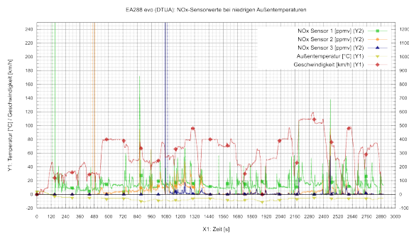
(a) Testfahrt bei -5 bis -11^{\circ}\text{C}
