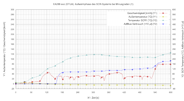
(a) Aufwärmzeit bei -5^{\circ}\text{C}
