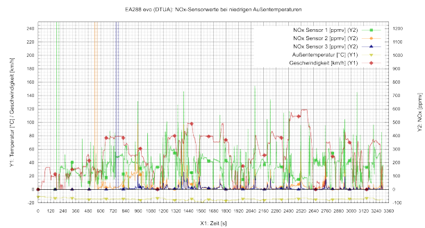
(b) Testfahrt bei -14 bis -19^{\circ}\text{C}
