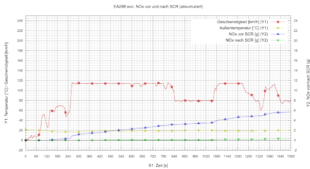
(a) \text{NOx} vor und nach SCR bei 120 km/h auf gerader Strecke
