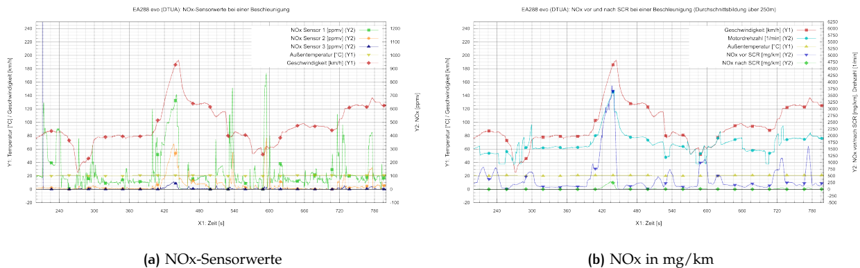
Abbildung 13: NO x -Werte bei einer Beschleunigung im 6. Gang
