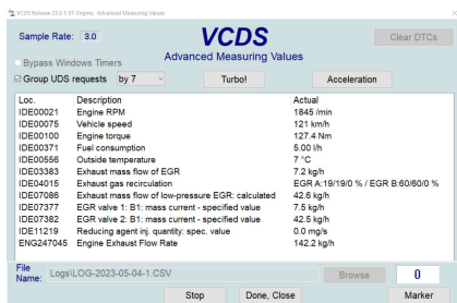
(a) AGR bei 120 km/h, niedrige Last
