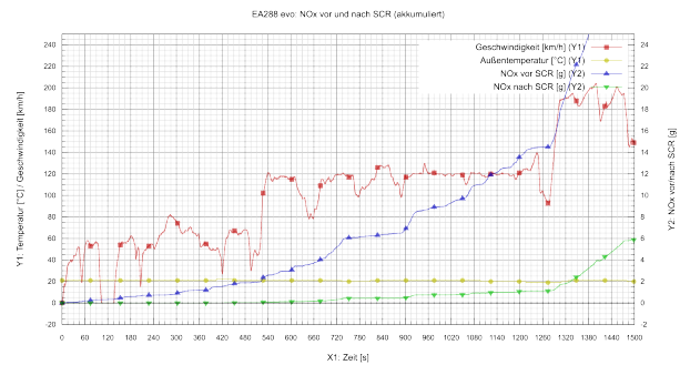
(b) \text{NOx} vor und nach SCR bei 120 km/h auf bergiger Strecke
