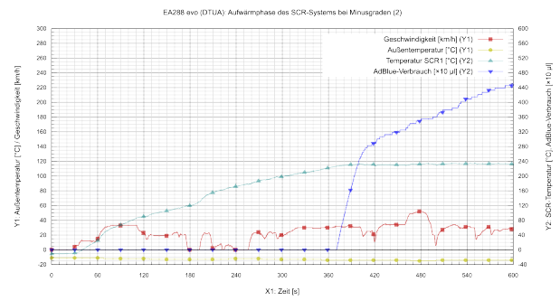
(b) Aufwärmzeit bei -14^{\circ}\text{C}
